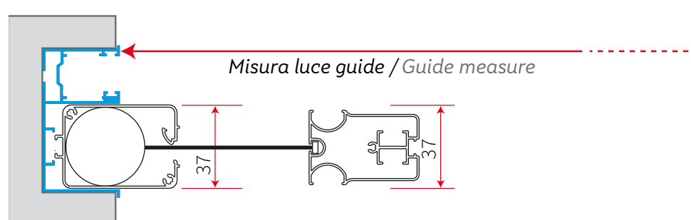
Sezione Orizzontale / Horizontal section
