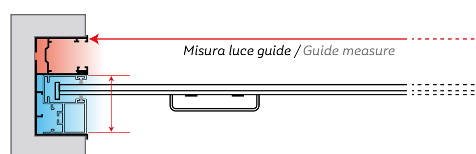
Sezione Orizzontale / Horizontal section
