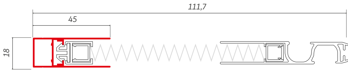
SISTEMA DI AGGANCIAMENTO FRONTALE / Frontal application
