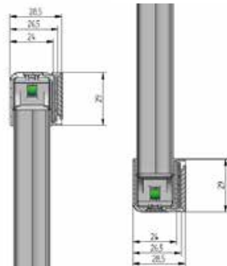
sezione verticale e frontale / vertical and frontal section
