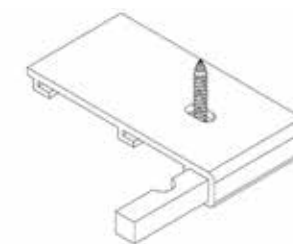
Attacco a soffitto Ceiling fastening
