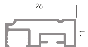
Profilo telaio / Frame profile
