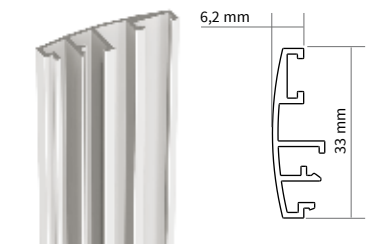
Z157 Profilo di battuta centrale Central frame profile
