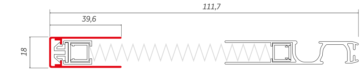
SISTEMA TRADIZIONALE / Standard application
