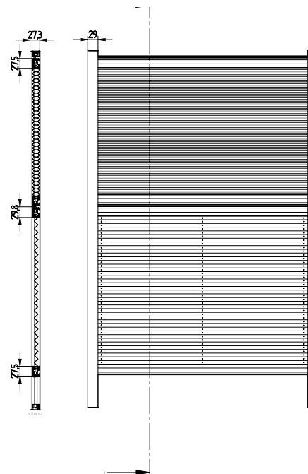
sezione verticale e frontale / vertical and frontal section
